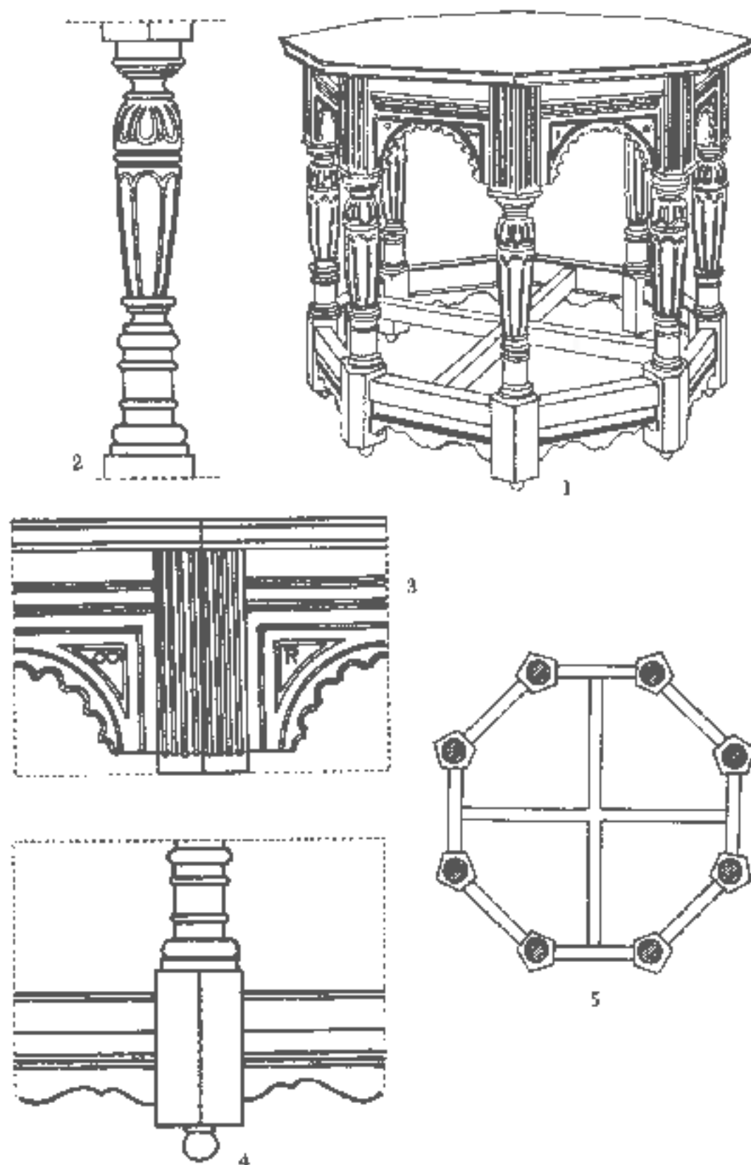
Lám. 59. — ESTILO TUDOR-ESTUARDO. 1. Característico mesa del final del reinado de Isabel: principios del siglo XVII. 2. Detalle ornamental de las patas. 3 y 4. Detalles ornamentales. 5. Plano. Colección particular.
