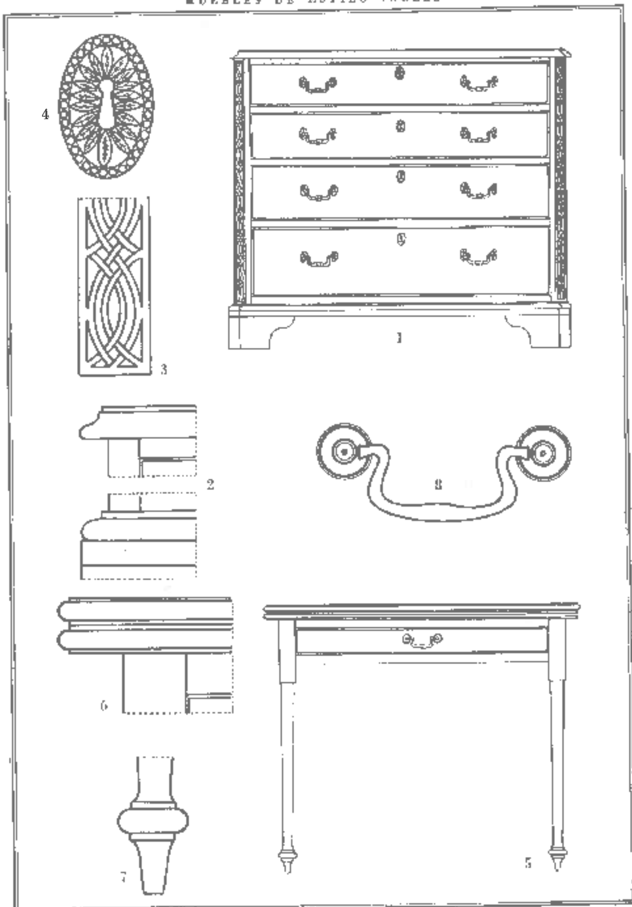
Lám. 403. ESTILO MENORQUÍN INGLÉS, 1. Chestón. 2. Detalle del maldurojo. 3. Detalle ornamental del mon-punto. 4. Frente. 5. Mesa. 6. Maldurojo al cubiero. 7. Detalle terminal de las patas. De la residencia de D. Francisco Mercedal Montauori, Mahón.
