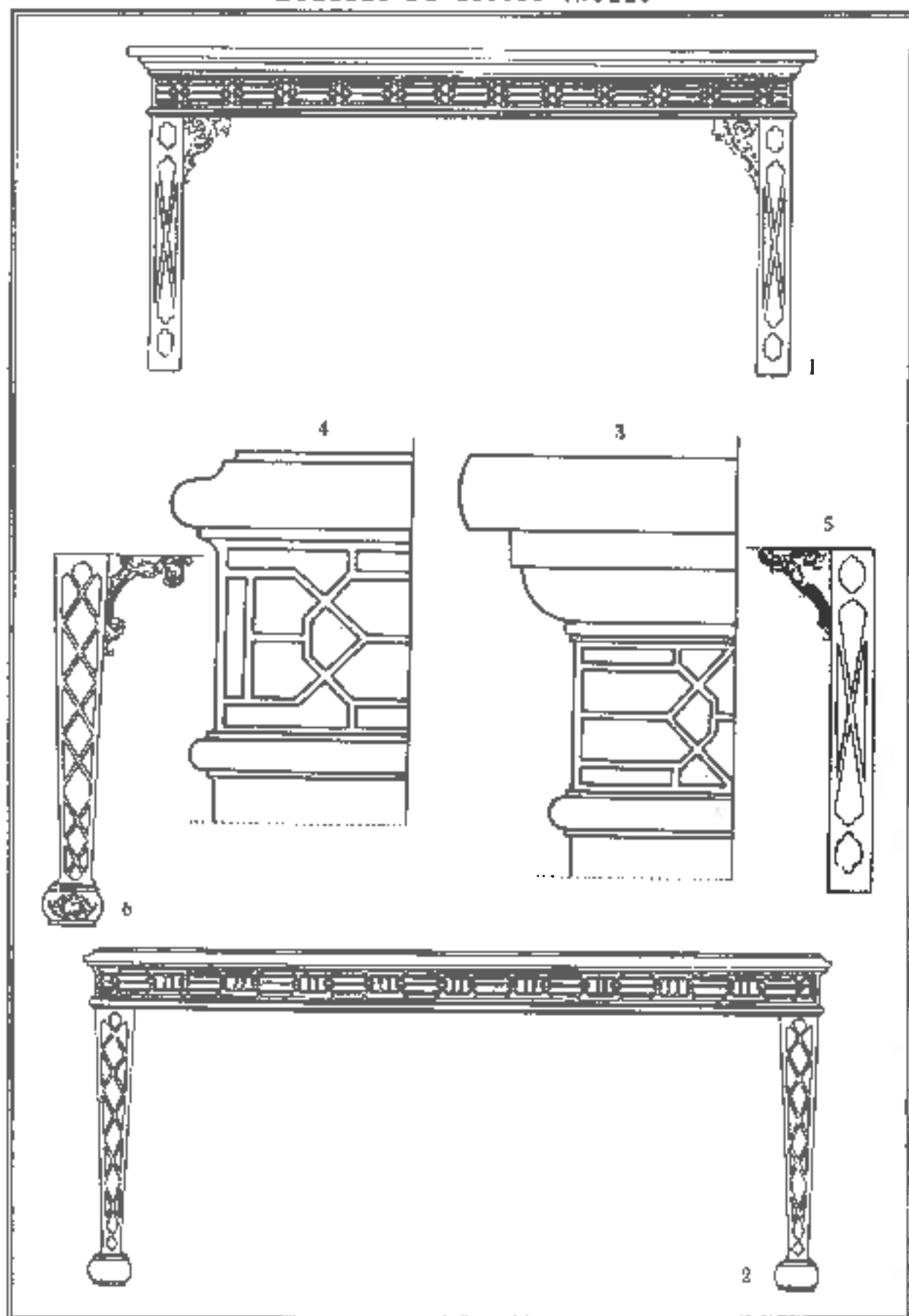
L. de M., 1745. — ESTILO CHIPPENDALE. 1 y 2. Mesas Chippendale con motivos chinos. 3. Moldura y friso de la primera. 4. Moldura y friso de la segunda. 5 y 6. Detalle de las patas respectivas. The Gentleman and Cabinet Maker's Guide. 7. Chippendale.
