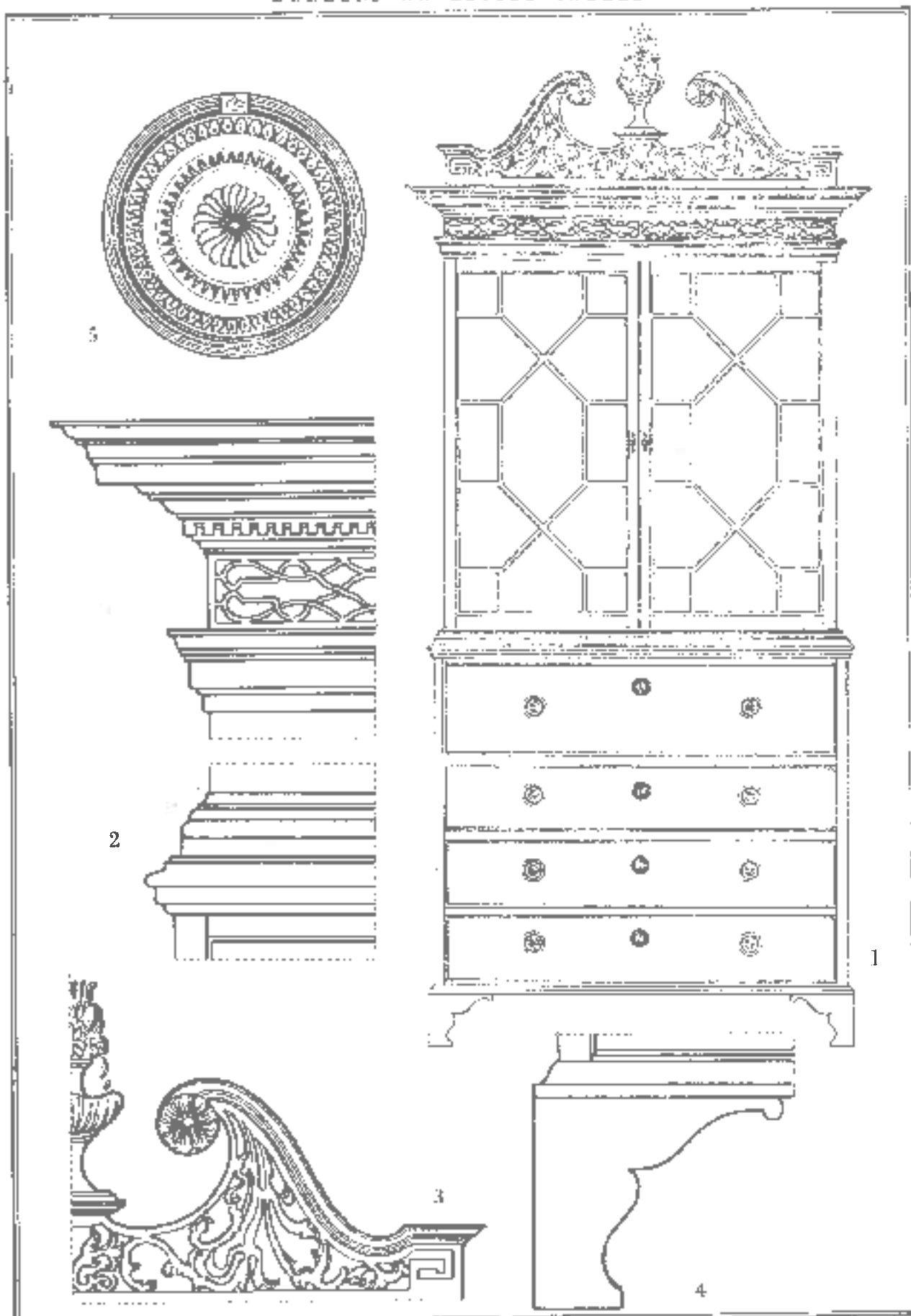
Lds. 571. — ESTILO MENORQUÍN INGLÉS. 1. Fábrica papíro. 2. Detalles ornamentales: entabl. friso y moldura. 3. Remate superior. 4. Perfil de la pata. 5. Tirador. De la residencia en D. a Juana Pons Guirart de Sukat, Mayor.
