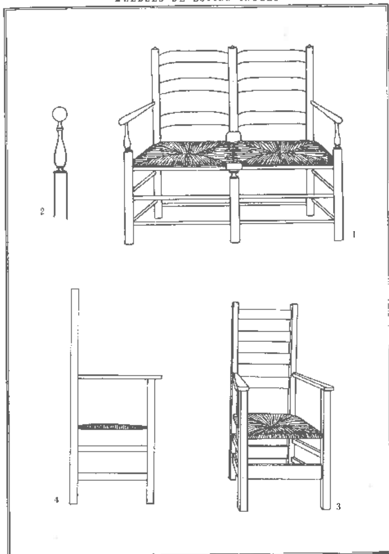
Lam. 294. ESTILO COLONIAL. 1. Sofá de factura Chippendale rural. 2. Detalle del soporte del brazo. Colección particular. 3. Silla de factura Chippendale rural. 4. Detalle de su estructura. Colección particular.
