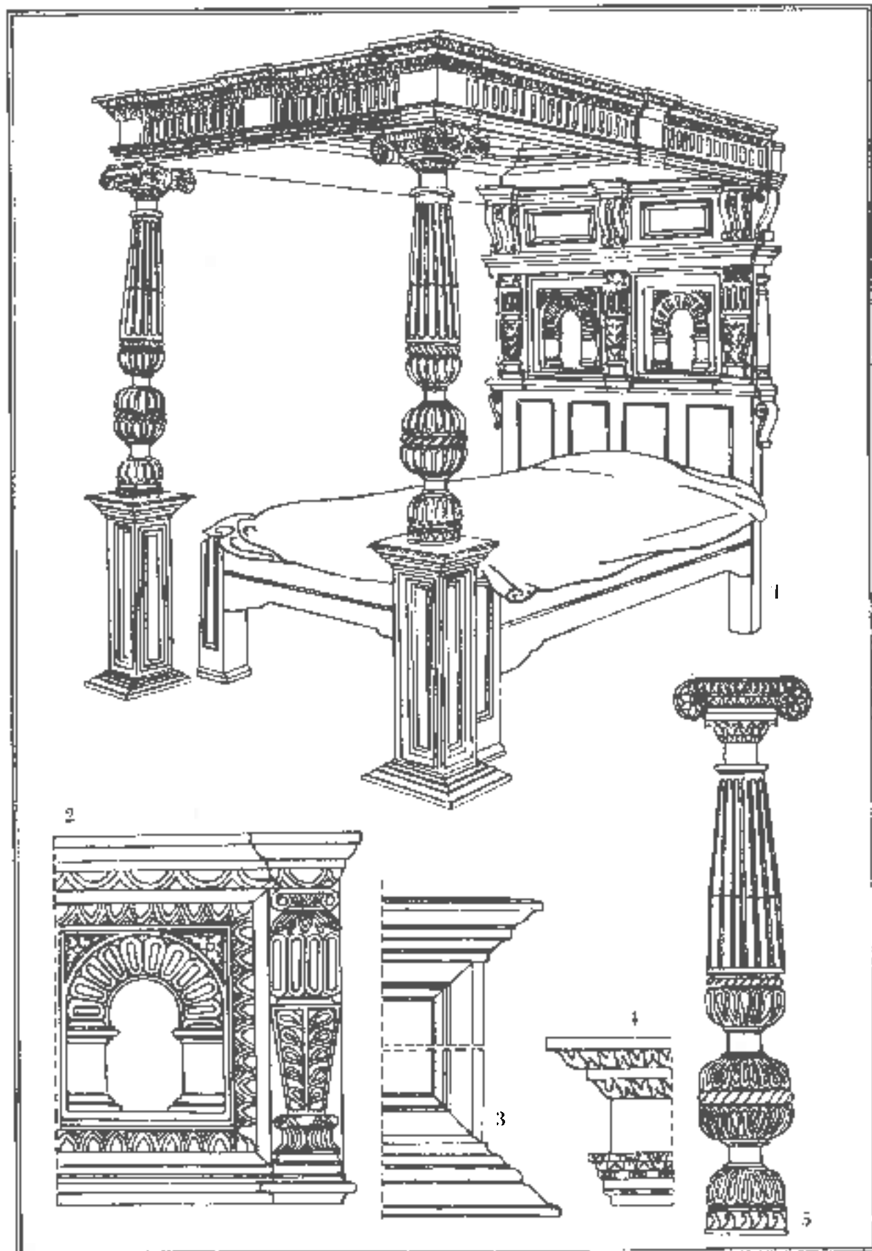
Lám. 78. ESTILO EL DOR-ESTUANDO. 1. Corner de cama, finales del siglo XVI. 2. Ornato ornamental de la cabecera. 3. Medidas de las pilastras del interior. 4. Ornamentación de las molduras del dintel. 5. Columna.
