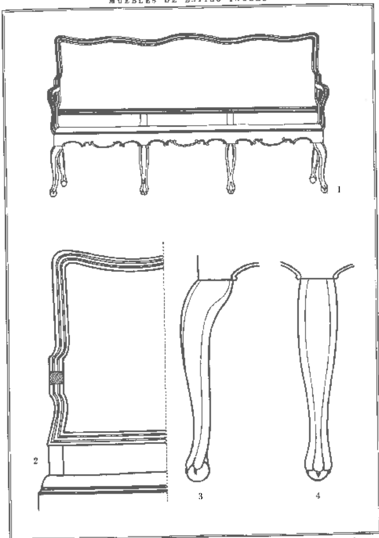
Lám. 323. — ESTILO MENDOTA EN INGLÉS. 1. Canapé. 2. Detalle del respaldo. 3. Pata terminal. 4. Pata central. De la residencia de D. Francisco Terrés Coll, Mahón
