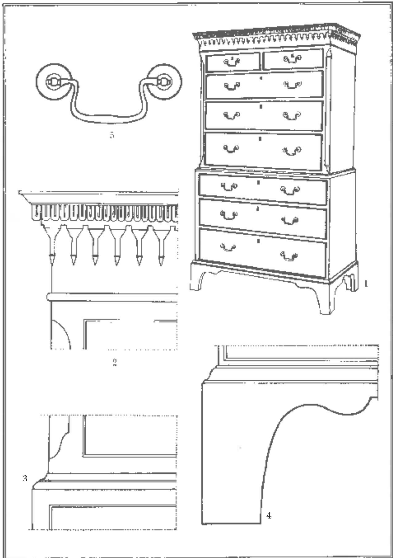
Lám. 204. — ESTILO CHIPPENDALE 1. Cónada alta de aspecto severo. 2. Detalle ornamental de la cornisa. 3. Moldura de la base del cuerpo superior. 4. Moldura inferior y pua. 5. Tirador. Colección particular
