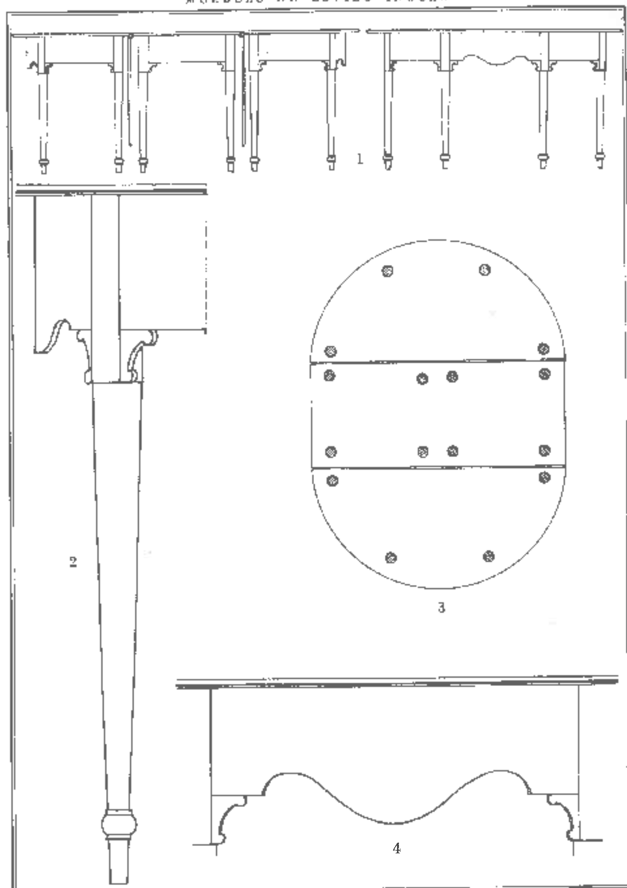
Lám. 422. — ESTILO MENDRQUIN INGLÉS. 1. Mesa formada por tres secciones. 2. Tornecado de las patas y moldura. 3. Planta. 4. Perfil superior. De la residencia señorial de los Condes de Torreblanca, Ciudadela.
