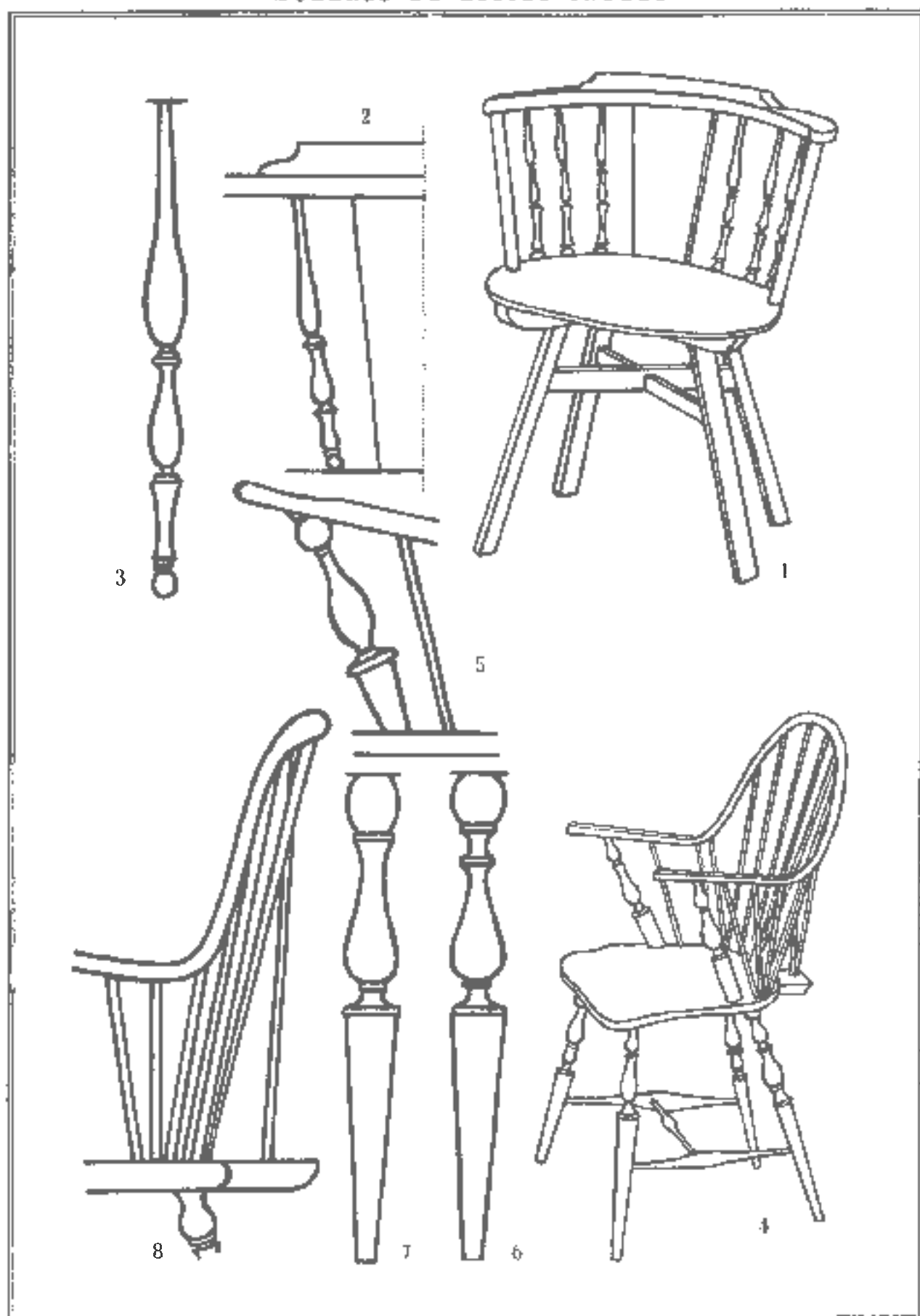
Lám. 305 — ESTILO COLONIAL. 1. Silla colonial típica. 2. Detalle del respaldo. 3. Tornavento de un huso. Colección particular. 4. Silla colonial típica. 5. Detalle terminal del huso. 6 y 7. Tornavientos de las patas. 8. Detalle de estructura del respaldo. Colección particular.
