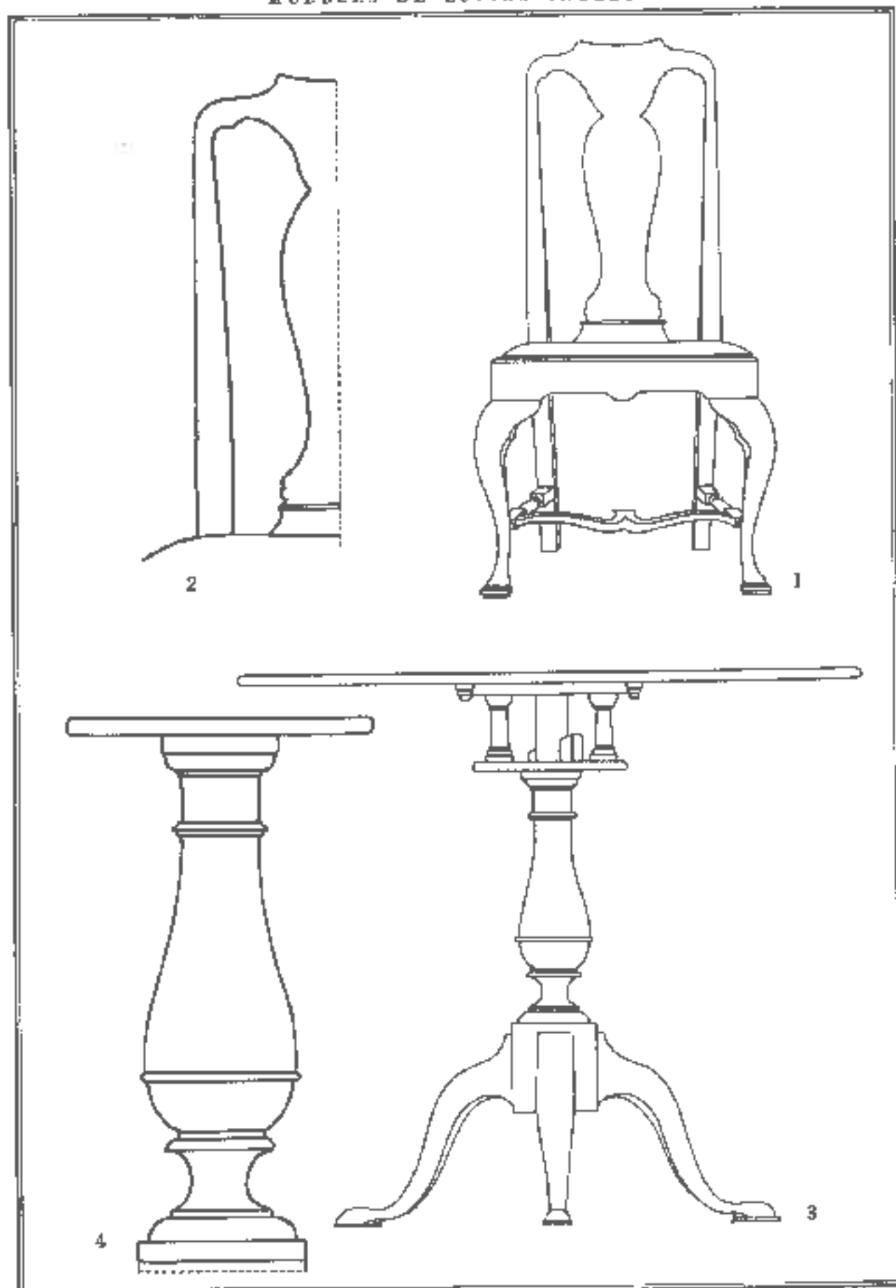
Lám. 331. — ESTILO MENORQUÍN INGLÉS 1. Silla de factura Reina Ana. 2. Detalle del respaldo. 3. Mesa de factura Reina Ana. 4. Tornavento de la columna central. De la residencia de D. Simón de Oliver Camet, Nación de Lluvia, Ciudadela.
