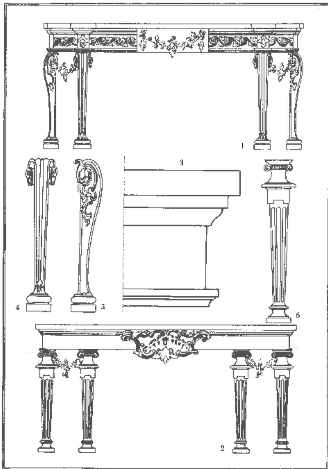
Lám. 196. — ESTILO CHIPPENDALE. 1 y 2. Mesas Chippendale fajosas. 3. Detalle de las molduras de la primera. 4 y 5. Detalles ornamentales de las patas de la primera. 6. Id. de la segunda. The Gentleman and Cabinet Maker's Guide. T. Chippendale
