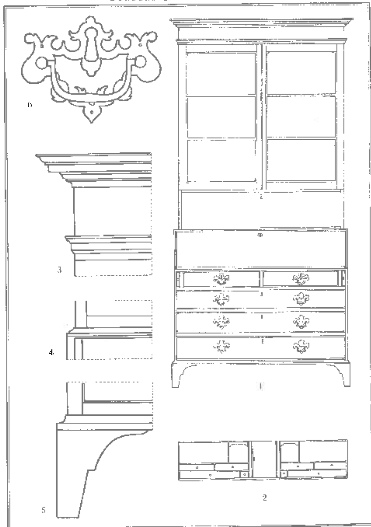
Lám. 323. ESTILO MENORQUÍN INGLÉS. 1. Librería (cupiro de dadas escritorio (acoplamiento ilógico). 2. De- tallo interior del cuerpo cubierto por la tapa reversible. 3, 4 y 5. Detalles ornamentales: cornisa, molduras y pila. 6. Trazador. He la residencia de D. Juan, Europa. Malaga
