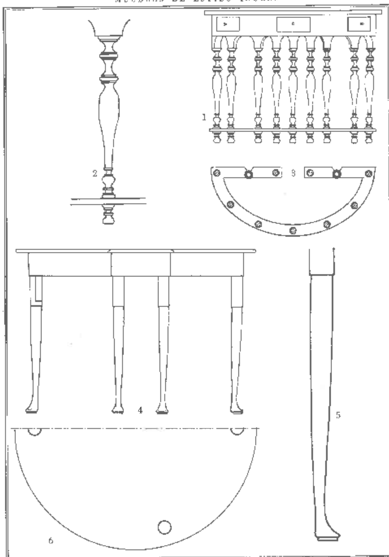
Lám. 123. ESTILO MENORQUÍN INGLÉS. 1. Mism. 2. Torneado de las patas. 3. Plancha. 4. Mesa de factura Reina Ana. 5. Torneado de las patas. 6. Plancha. De la tridectria reducida de las London de Torresaur. Ciudadela.
