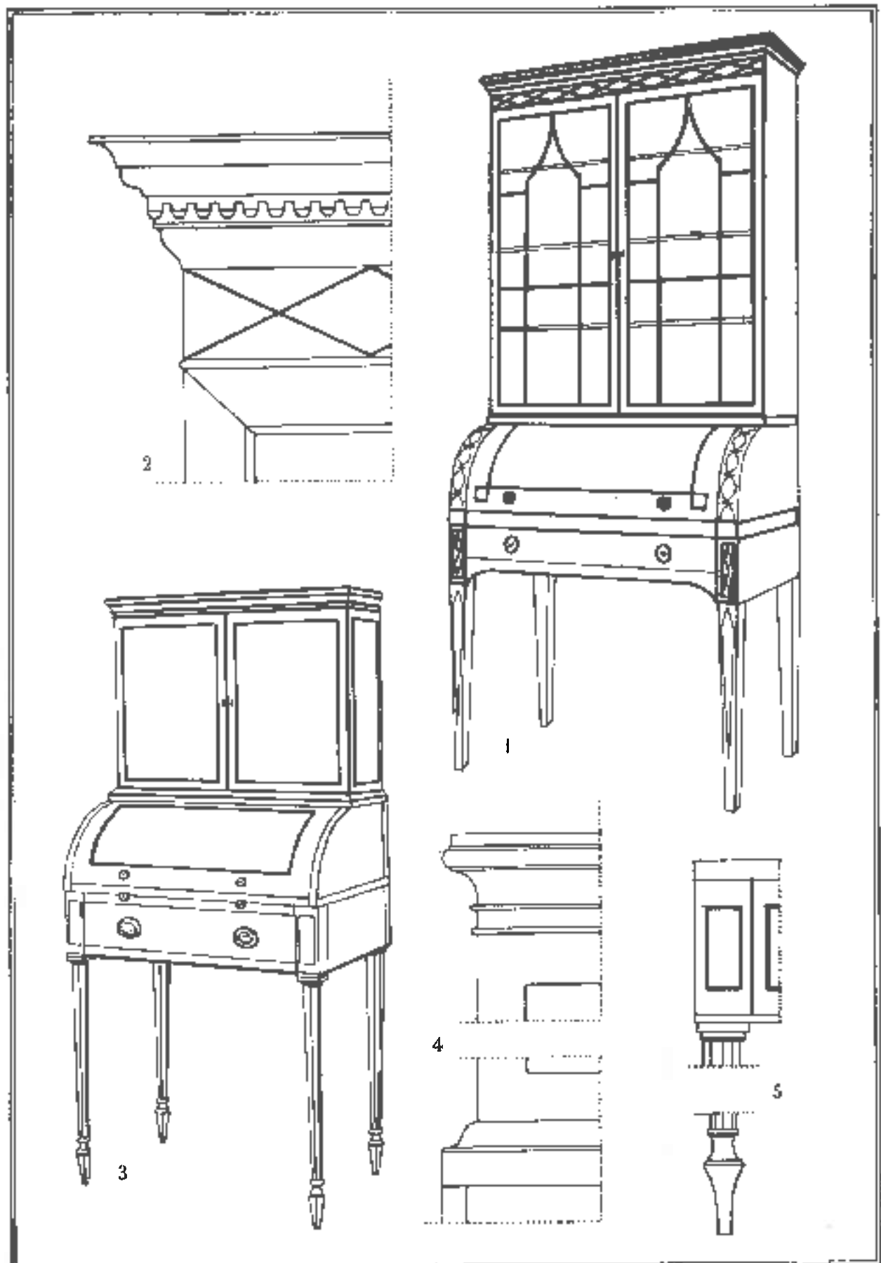
Lam. 372. ESTILO SHERATON. 1. Escritorio Sheraton. 2. Detalle de la cornisa y ángulo superior. Victoria and Albert Museum. — 3. Escritorio Sheraton. 4. Moldura del cuerpo superior. 5. Detalle de la pata perteneciente a M. George Smeat de West Wickham, realizado de Kent.
