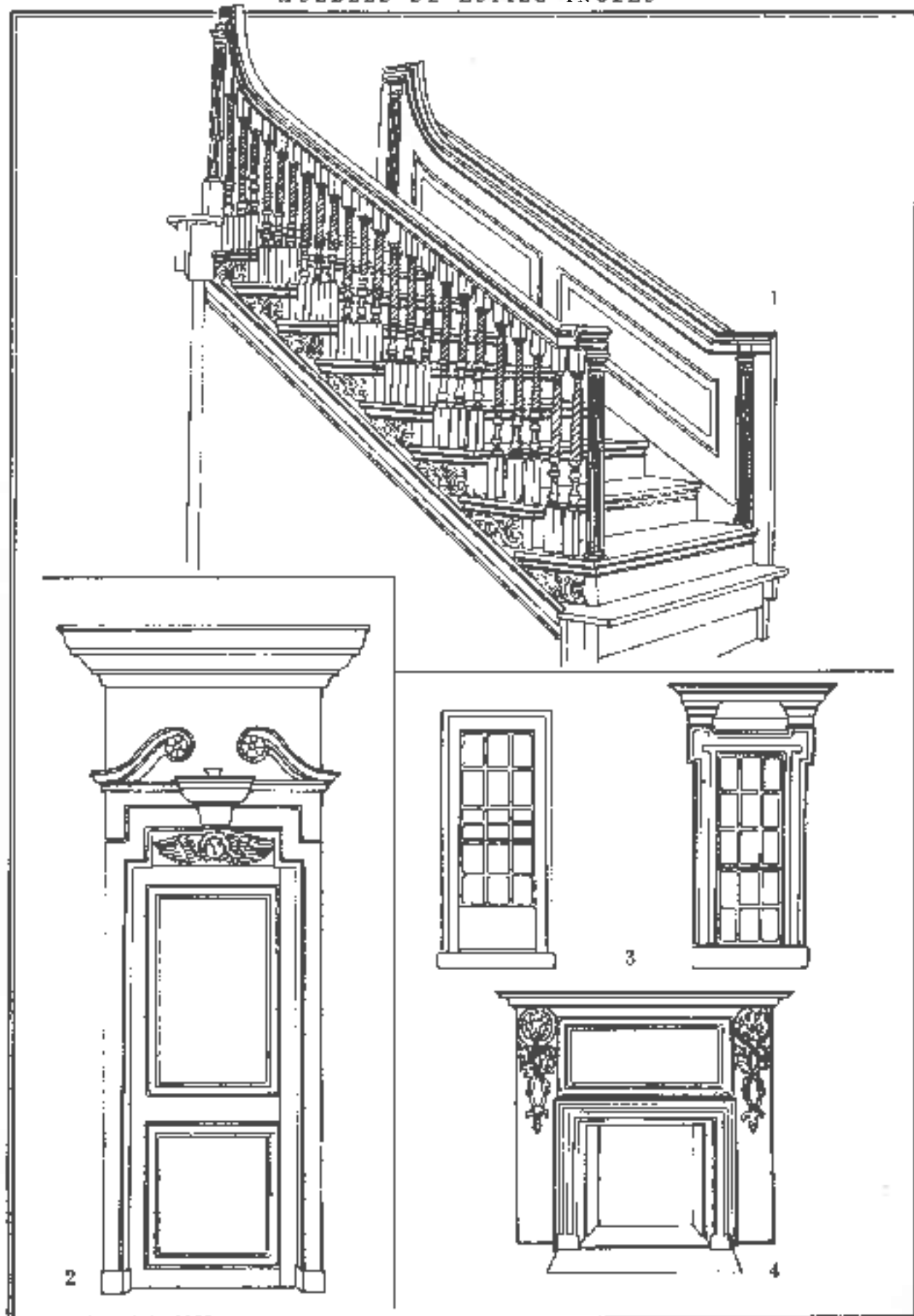
Lam. II -- ESTILO REINA ANA. 1. Porción de escalera de madera de pino acopiada; finales del siglo XVII. Castelnau House, Chertok. 2. Puerta de habitación. Clifford's Inn, Londres. 3. Ventanas jorginadas. La primera de la Casa del Com. Chertok. La segunda de Raynham Hall, Norfolk. 4. Chimenea de Grindling Gibbon. Palacio de Hampton Court.
