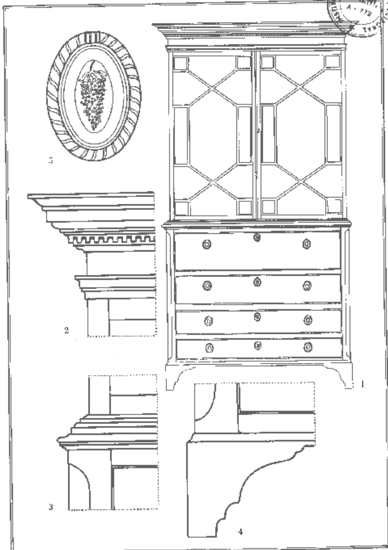
Tabl. 391. — ESTILO MENDOQUÍN INGLÉS. 1. Armario inglés. 2, 3 y 4. Detalles ornamentales: cornisa, moldura y perfil de la pata. 5. Tirador. De la residencia de D. a Juana Guinart de Salort, Alayor.
