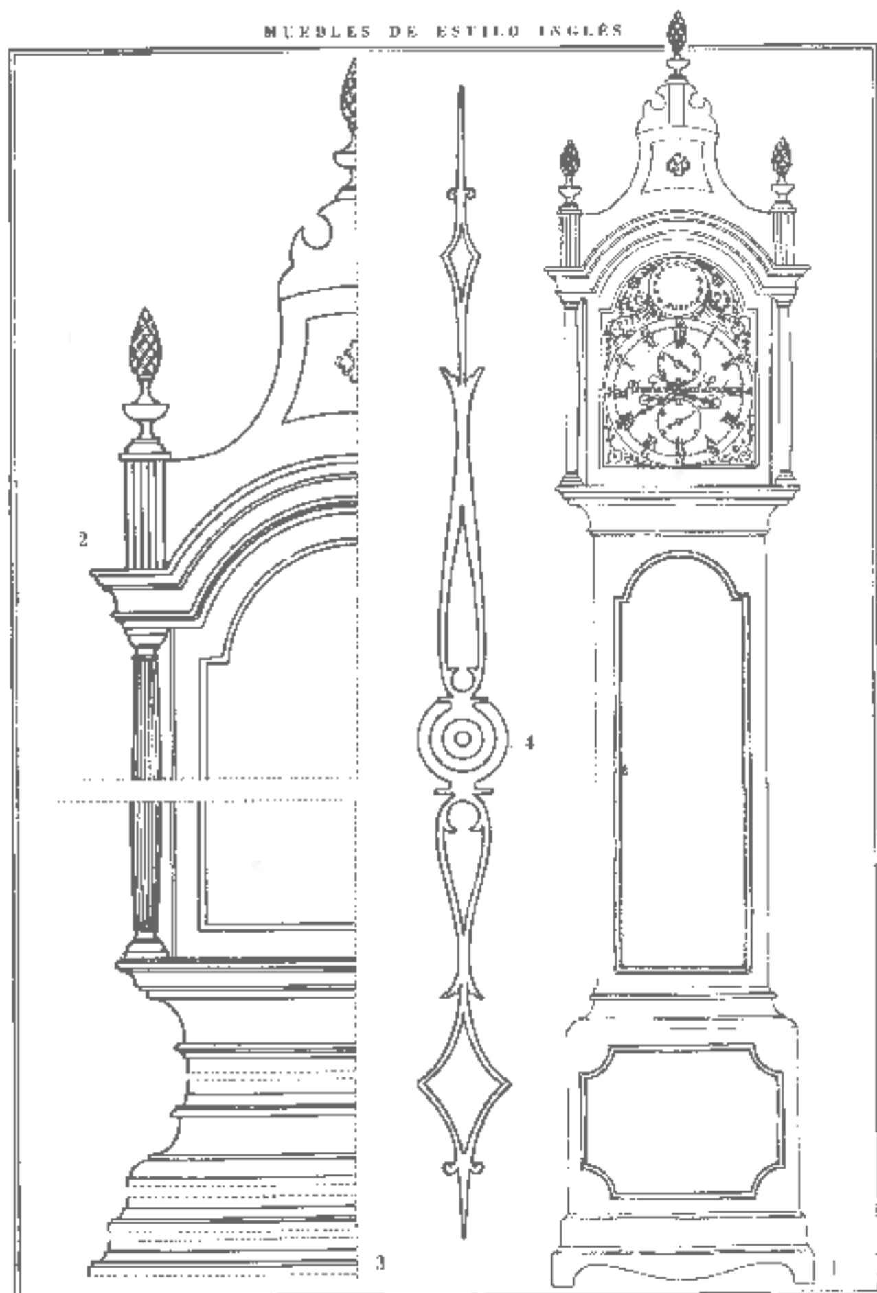
Lám. 412 ESTILO MENORQUÍN INGLÉS. 1. Caja de reloj. 2 y 3. Detalles ornamentales: remate, cornisa, columna y molduras. 4. Manecillas. En la residencia del Barón de Bimmarsten, D. Espiridión Rodríguez de la Tuxina Mahón.
