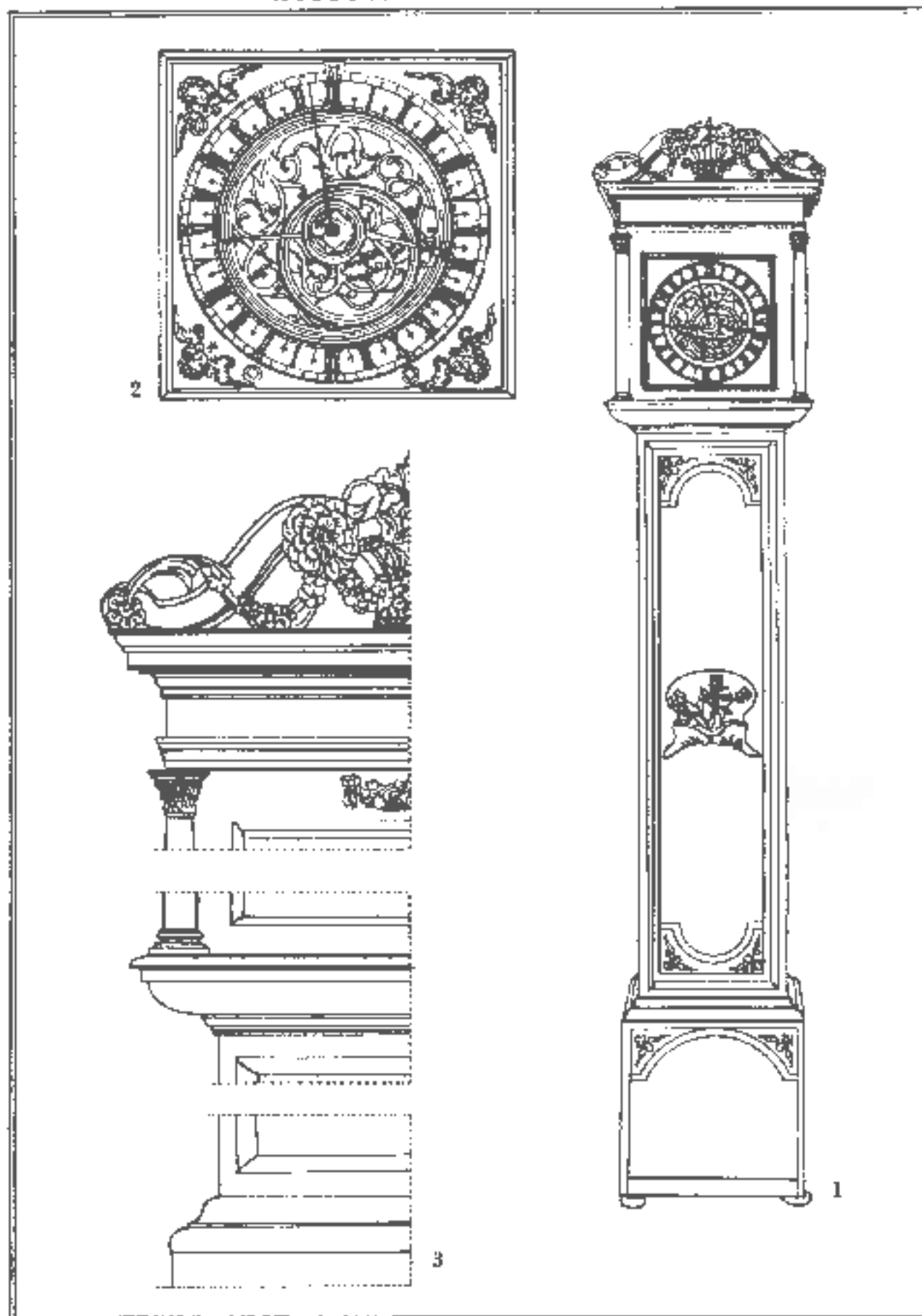
Lám. 85. - ESTILO TUDOR-ESTUARDO. 1. Caja de reloj del siglo XVII. 2. Esfera de urticumero horas. 3. Detalle de molduras y remate. Colección de S. E. Prestige
