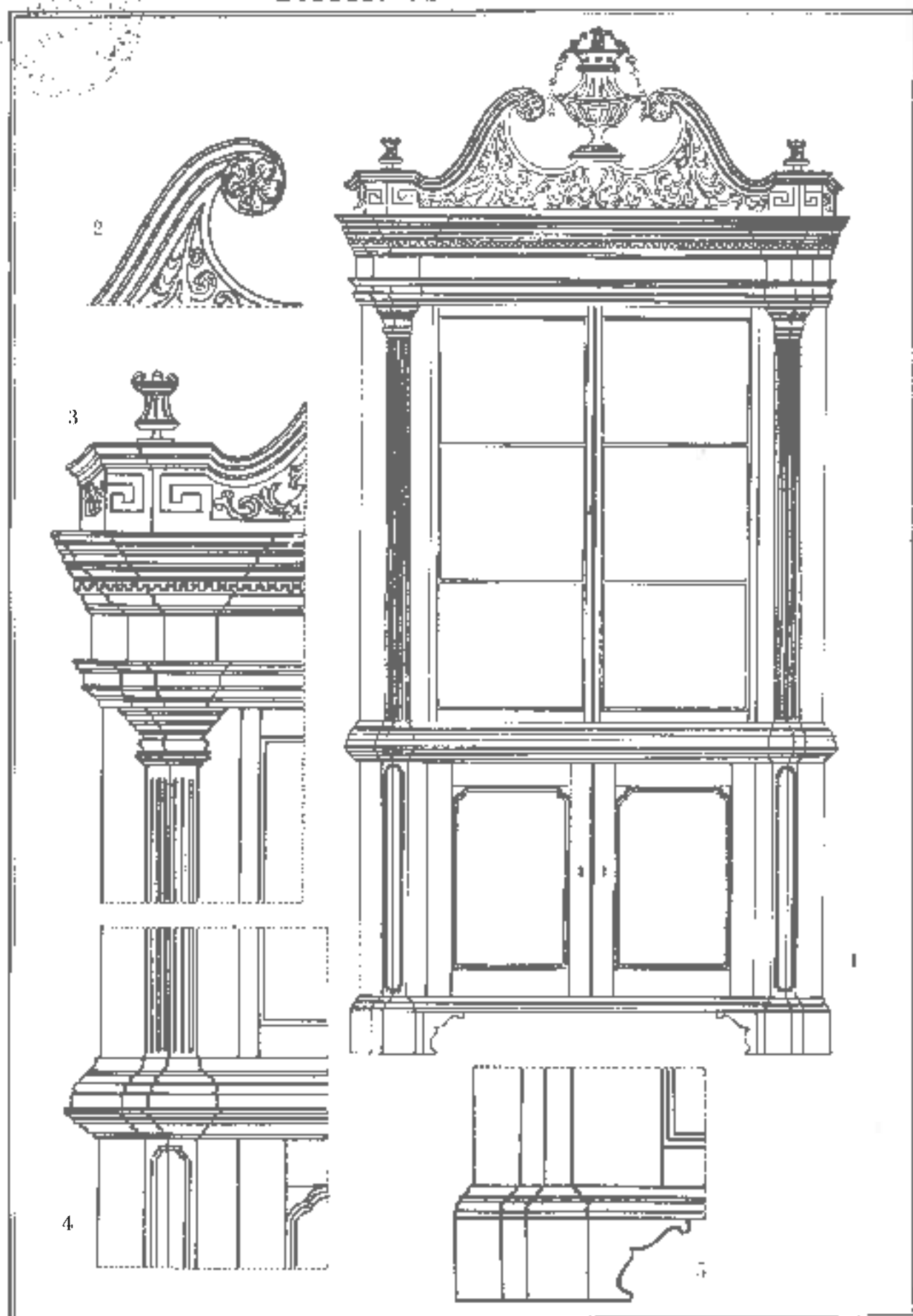
Lám. 386. - ESTILO MINORQUÍN INGLÉS. 1. Armario curro de estorgado moldureja. 2. Detalle del remate. 3, 4 y 5. Detalles ornamentales: remate, molduras, columnas y para. De la residencia de D. a María Antonia Felín, Vda. de Olives. Mahón.
