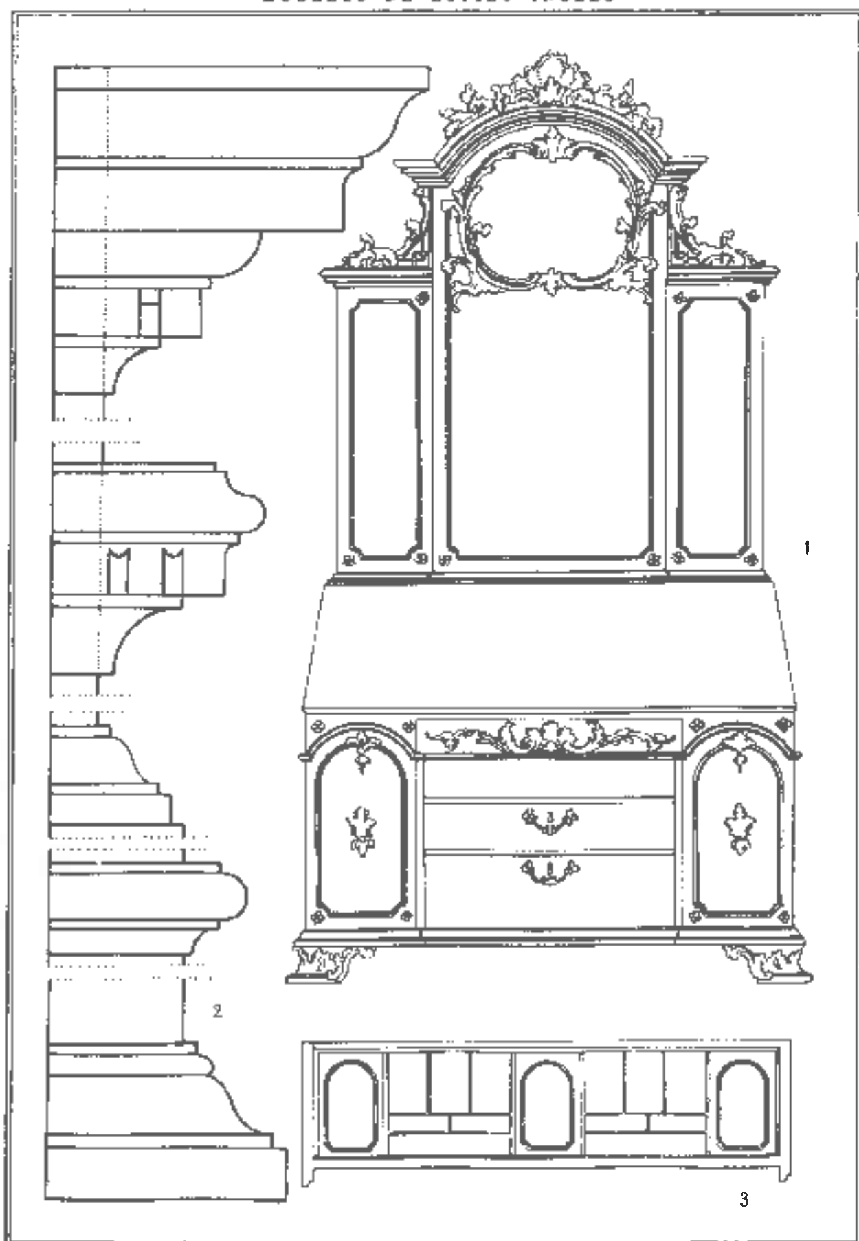
Lám. 212.— ESTILO CHIPPENDALE. 1. Librería escritorio dibujada por Chippendale. 2. Detalle de cornisas y molduras. 3. Id. del cuerpo inferior de la librería, cubierto por la tapa reversible. The Gentleman and Cabinet Maker's Guide. T. Chippendale
