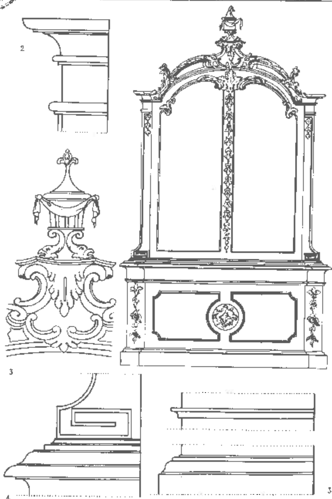
Lám. 216. - ESTILO CHIPPENDALE. 1. Librería dibujada por Chippendale. 2. Cernisa. 3. Remate superior. 4. Base y moldura inferior del cuerpo de la librería. 5. Molduras del cuerpo inferior. The Gentleman and Cabinet Maker's Guide. T. Chippendale
